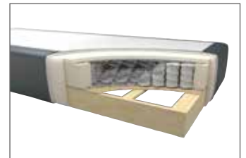
Taschenfederkern
