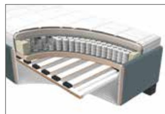
2-Schicht-Aufbau
